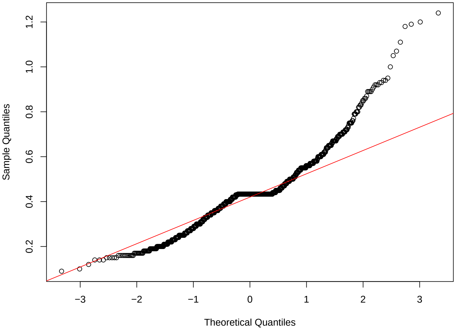
Q-Q Plot: lipids5
